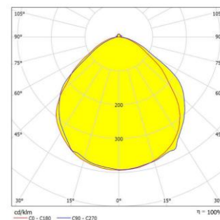
Distribuția Luminanței
