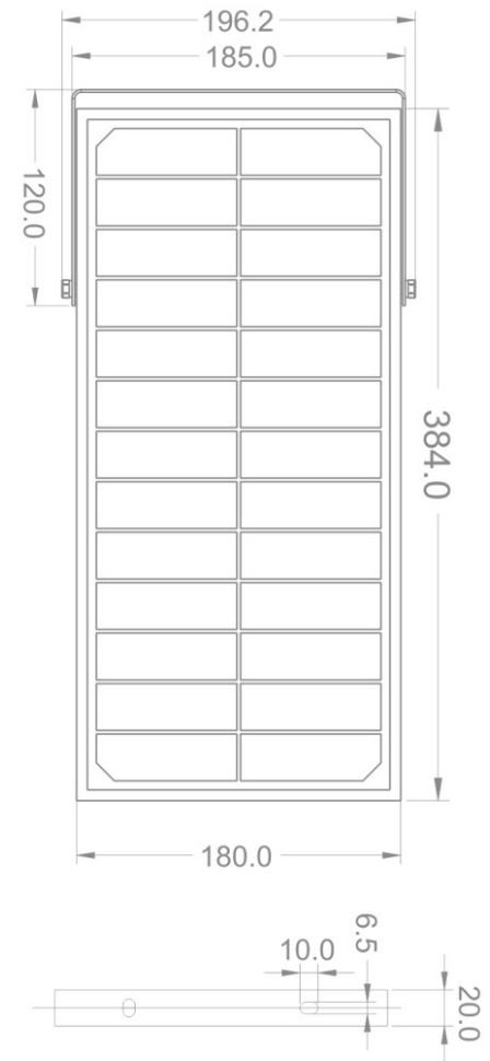
PANOUL SOLAR
